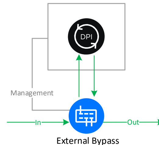
Внешний bypass любого производителя, управляемый SKAT DPI
